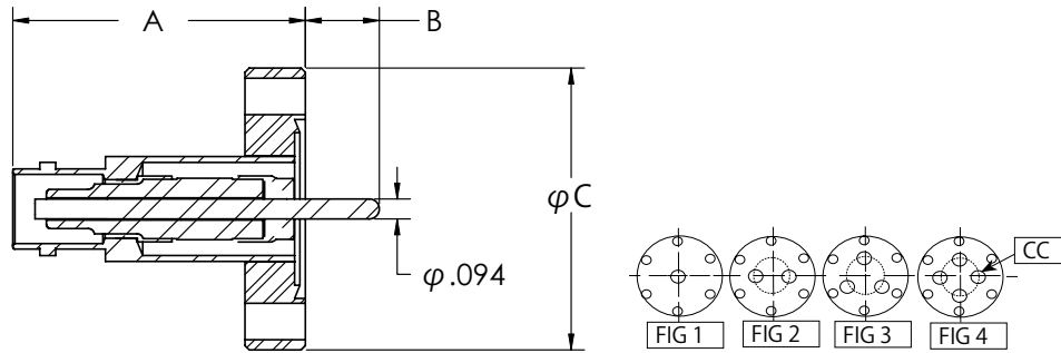
ボルト穴と端子の相対位置は参考です。
